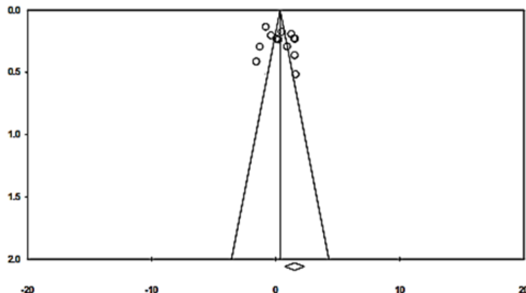
شکل ۱. نمودار فائل (قیفی)
